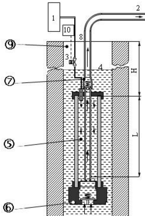
Figura 1. Croquis de la bomba neumática simple. Donde: (1) Fuente de aire comprimido; (2) Salida de agua; (3) Electroválvula AB; (4) Nivel de agua; (5) Cámara; (6) Válvula de retención TR1; (7) Válvula de retención TR2; (8) Nivel del suelo; (9) Perforación; (10) Controlador de tiempos lógico programable (CTLP - Control automático de la electroválvula AB).
