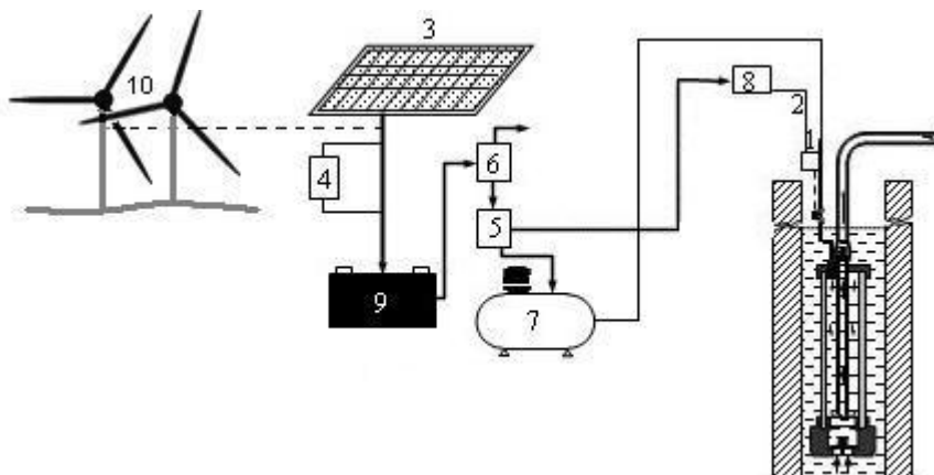
FIGURA 3. Sistema completo para la extracción de agua mediante energías alternativas. Donde: (1) electroválvula de aire comprimido; (2) circuito eléctrico de comando de electroválvulas; (3) paneles solares, (4) regulador de voltaje; (5) inversor de corriente CC/AC;
