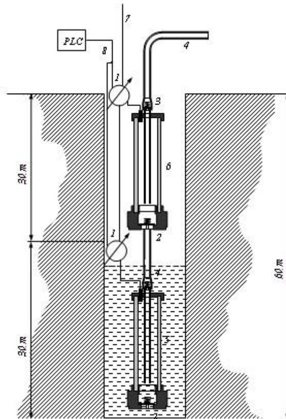
Figura 2. Corte esquemático del sistema de bombeo de agua mediante aire comprimido de dos etapas. Donde: (1) electroválvula de aire comprimido; (2) válvula de retención 2 1/2"; (3) válvula de retención 3/4"; (4) caño 3/4"; (5) cámara 1; (6) cámara 2; (7) cañería 3/4" de aire comprimido; (8) circuito eléctrico de comando de electroválvulas
