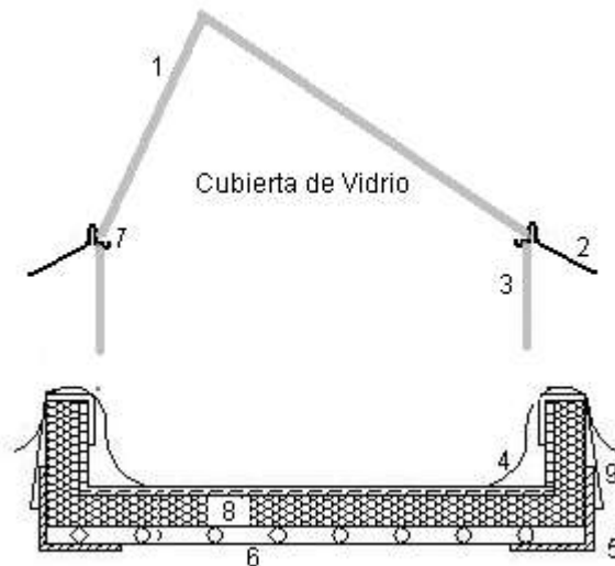
Figura 1: Corte del destilador solar de batea liviana: 1 cubierta de vidrio – 2 Perfiles de chapa acero inoxidable que sostiene la cubierta de vidrio. 3 – soportes de vidrio que apoyan sobre el fondo de la batea cerrando el receptáculo. 4 Polietileno negro. 5 Marco de hierro ángulo. 6 malla de acero de construcción. – 7 canales de agua destilada. 8 aislante térmico (Poliestireno expandido mas cartón corrugado) – 9 perfiles de chapa galvanizada que cierran la batea.
